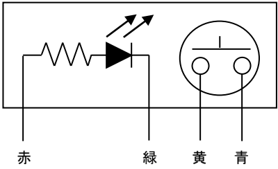
内部回路
